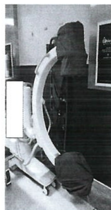
ภาพผ้าคลุมตัวรับภาพและผ้าคลุมหลอดเอกซเรย์เมื่อใส่กับเครื่อง
